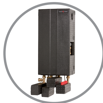
Termix VMTD Mini opbl. ISO m/påbygget fordelerrør
