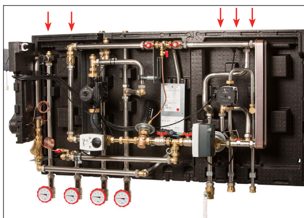
Rør monteres. Fjernvarmerør ombyttes.
