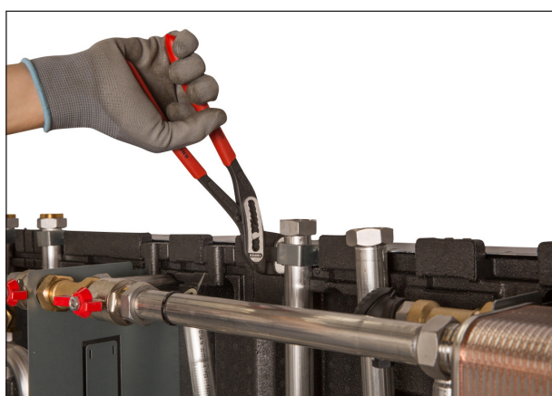
U-bøjler monteres.
