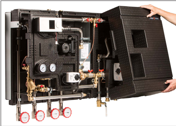
Isoleringscover monteres for brugsvandenheden.
